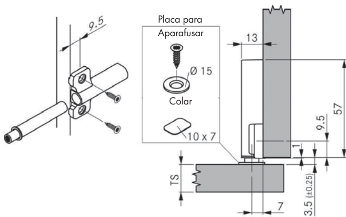
Adaptador batente
