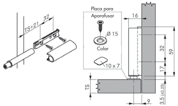
Adaptador reto
