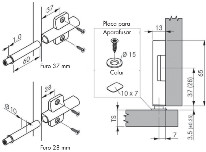
Adaptador multifuro
