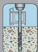
Bohrloch herstellen
