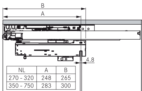
Position Synchronisationsstange
